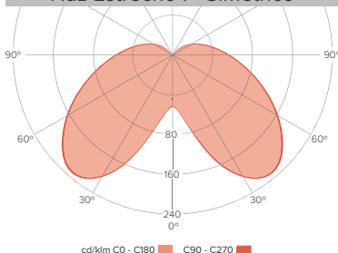
Haz Estrecho I - Simétrico
