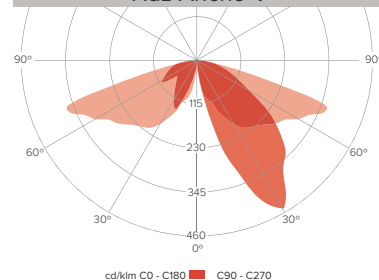
Haz Ancho V
